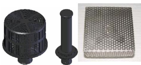
Всасывающий фильтр Труба сброса
